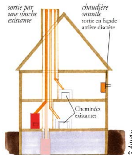
Chaudière dans la cave ou mieux, dans l'habitation
